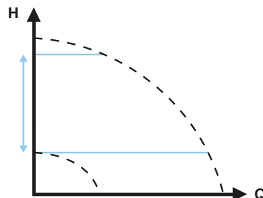
Obr. 24 Nastavení křivky konstantního tlaku
