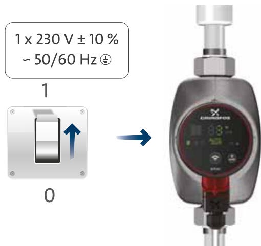
Obr. 6 Spouštění čerpadla
