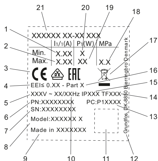
Obr. 11 Typový štítek
